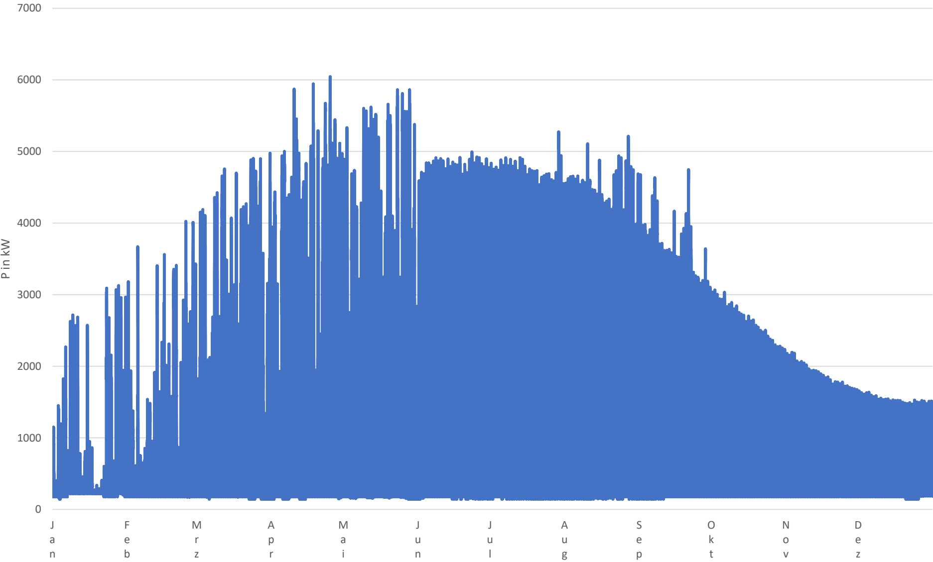
Einspeisung Niederspannung im Jahr 2024
