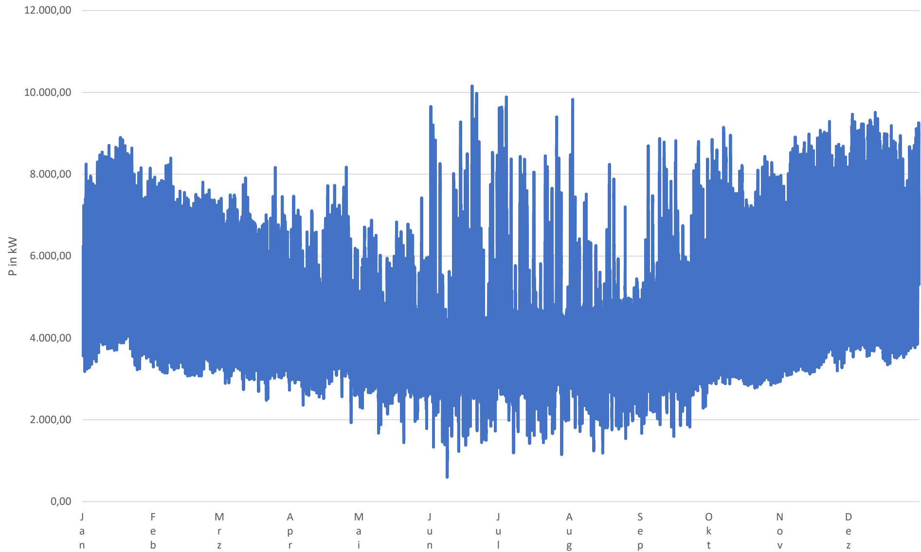
Summenlast der nicht leistungsgemessenen Kunden im Jahr 2024
